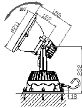
A: 30.0724 HIT 灯具尺寸图
